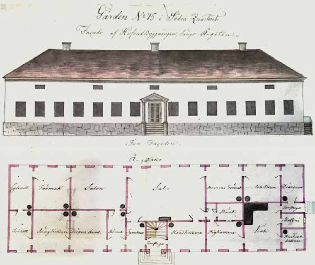
Eteläkorttelin tontilla 75 sijainneen af Schulténien talon sisäpihan julkisivu ja pohjapiirros. Rakennuksen suunnitteli professori Gabriel Bonsdorff vuonna 1813.
