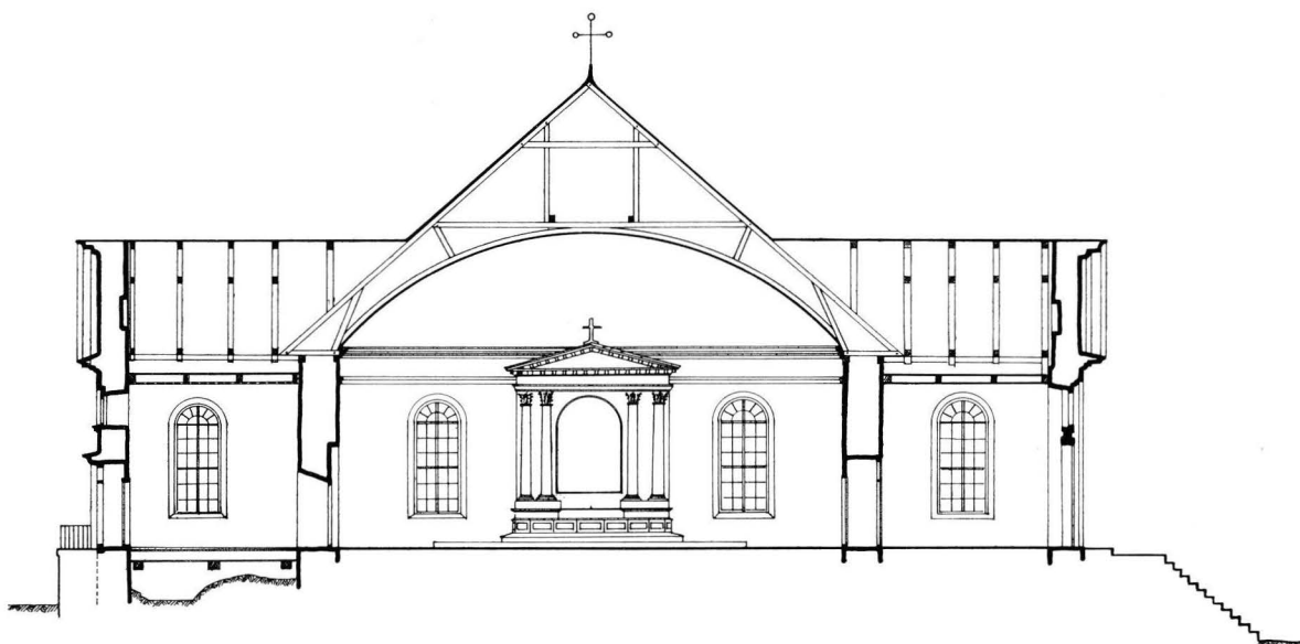
27. KIRKON ITÄSUUNTAINEN POIKITTAISLEIKKAUS, 1:300. Tvärssnitt av kyrkan mot öster, 1:300.
