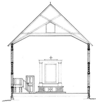
6. KIRKON ITÄSUUNTAINEN POIKITTÄISLEIKKAUS, 1:300. Tvärssnitt av kyrkan mot öster, 1:300.
