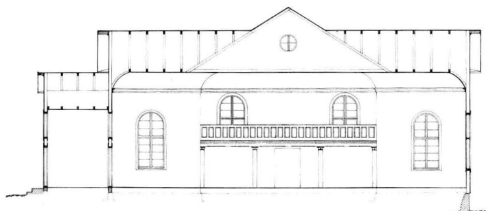
6. KIRKON LÄNSISUUNTAINEN POIKITTÄISLEIKKAUS, 1:300. Tvärsnitt av kyrkan mot väster, 1:300.
