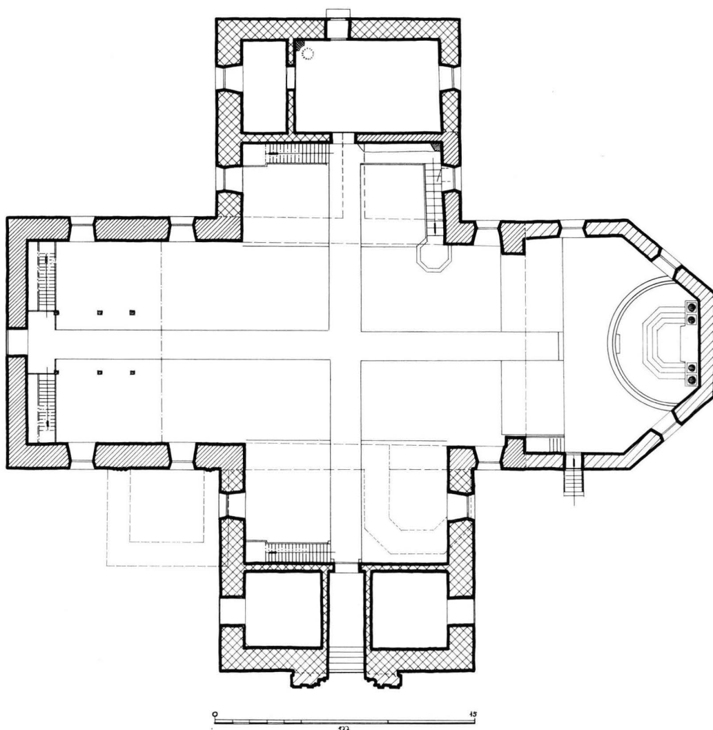
14. KIRKON POHJAPIIRROS, 1:300. Plan av kyrkan, 1:300.
