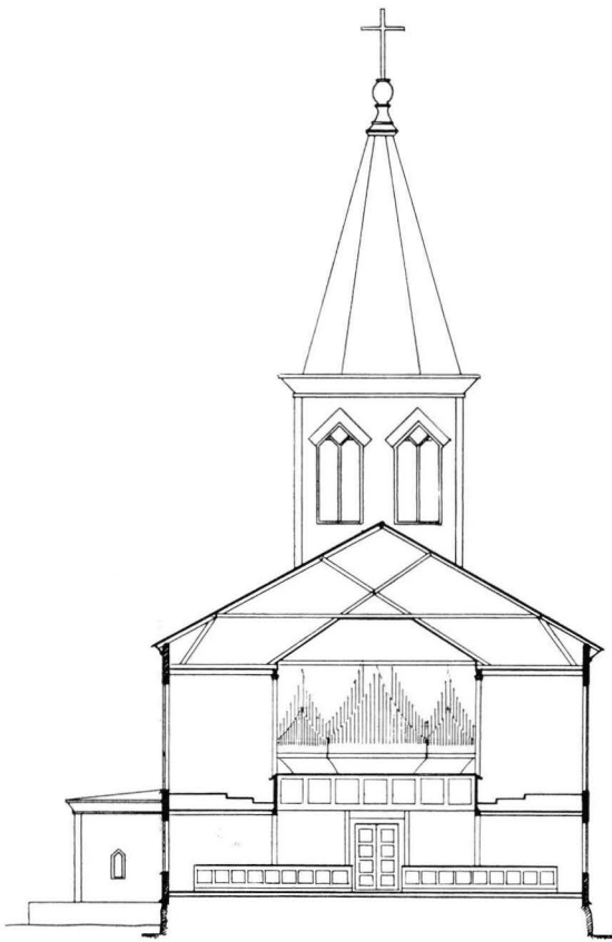
9. KIRKON LÄNSISUUNTAINEN POIKITTAISLEIKKAUS, 1:300. Tvårsnitt av kyrkan mot väster, 1:300.
