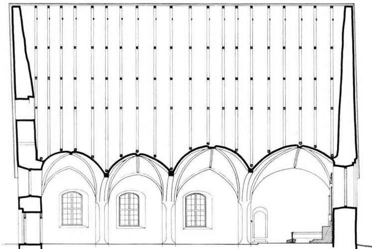
8. KIRKON POHJOISSUUNTAINEN PITKITTÄISLEIKKAUS, 1:300. Längdsnitt av kyrkan mot norr, 1:300.
