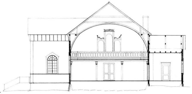
9. KIRKON LÄNSISUUNTAINEN POIKITTÄISLEIKKAUS, 1:300.
