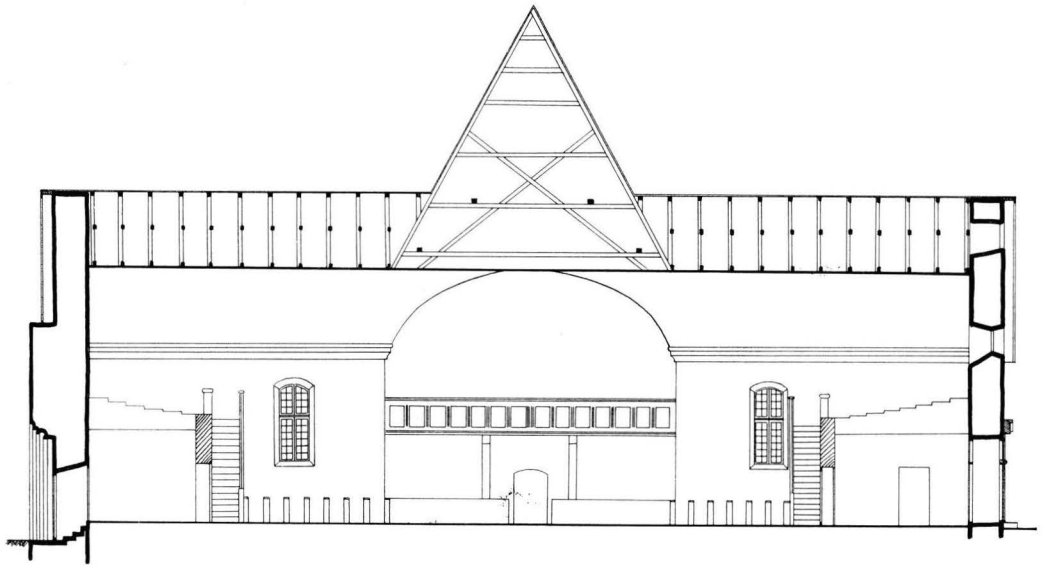
15. KIRKON LÄNSISUUNTAINEN POIKITTÄISLEIKKAUS, 1:300. Tvärnsnitt av kyrkan mot väster, 1:300.
