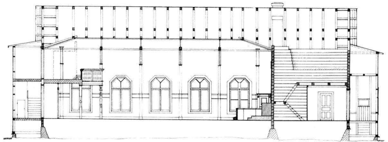
46. POHJOISSUUNTAINEN PITKITTÄISLEIKKAUS, 1:300. Längdsnitt mot norr, 1:300.
