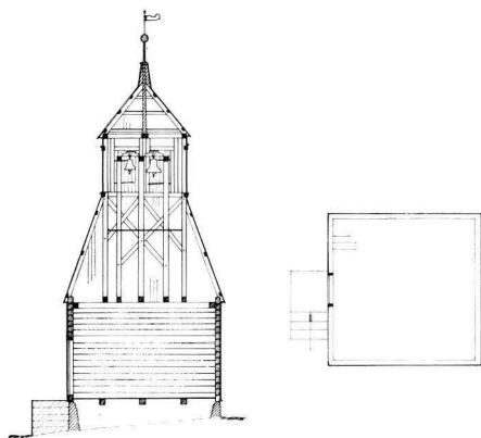
4. TAPULIN PYSTYLEIKKAUS JA POHJA, 1:300. Snitt och plan av stapeln, 1:300.
