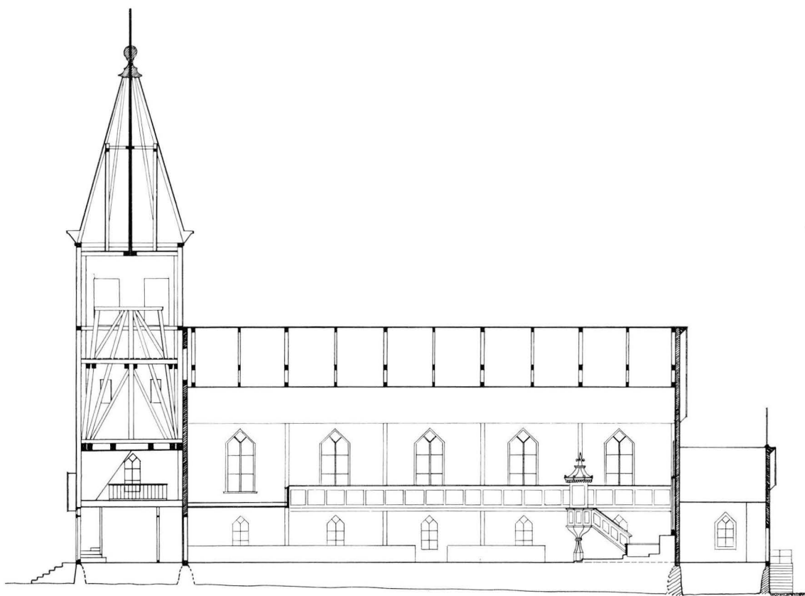
7. KIRKON POHJOISSUUNTAINEN PITKITTÄISLEIKKAUS, 1:300. Längdsnitt av kyrkan mot norr, 1:300.
