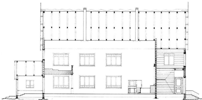
5. KIRKON ETELÄSUUNTAINEN PITKITTÄISLEIKKAUS, 1:300. Längdsnitt av kyrkan mot söder, 1:300.
