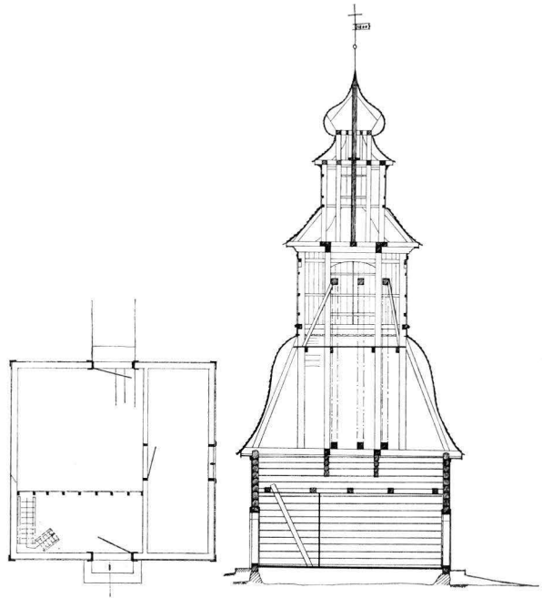
3. TAPULIN PYSTYLEIKKAUS JA POHJA, 1:300. Snitt och plan av stapeln, 1:300.
