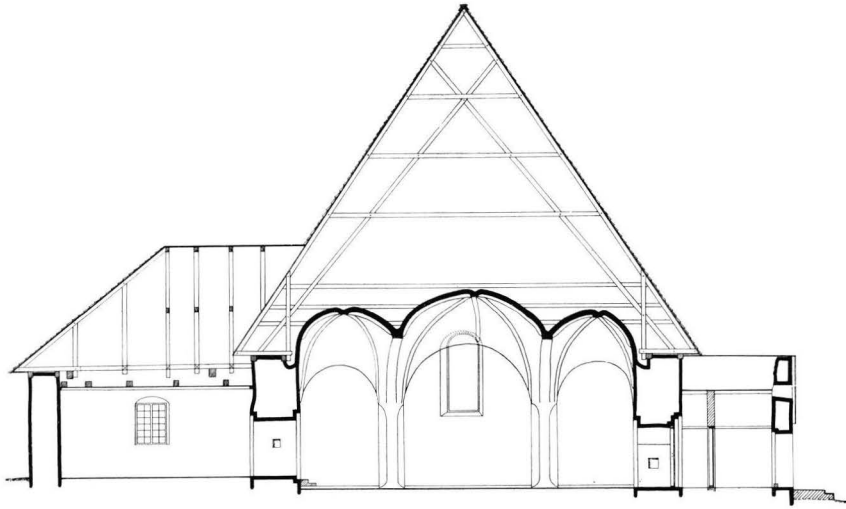
7. KIRKON ITÄSUUNTAINEN POIKITTÄISLEIKKAUS, 1:300. Tvärssnitt av kyrkan mot öster, 1:300.
