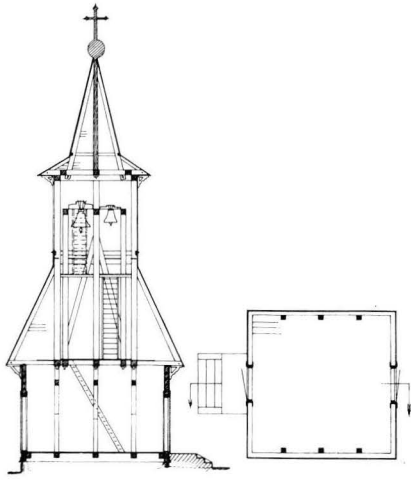
3. KELLOTAPULIN PYSTYLEIKKAUS JA POHJA, 1:300. Snitt och plan av klockstapeln, 1:300.
