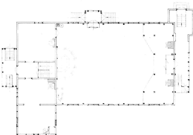
48. POHJAPIIRROS, 1:300. Plan, 1:300.
