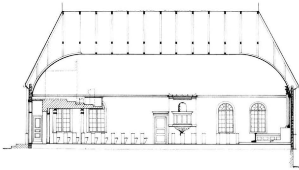
7. KIRKON POHJOISSUUNTAINEN PITKITTÄISLEIKKAUS, 1:300.
