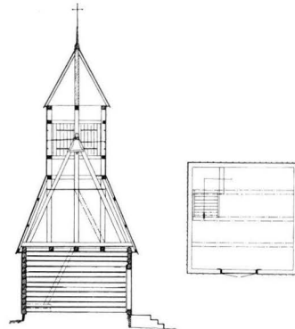
3. TAPULIN PYSTYLEIKKAUS JA POHJAPIIRROS, 1:300. Snitt samt plan av klockstapel, 1:300.
