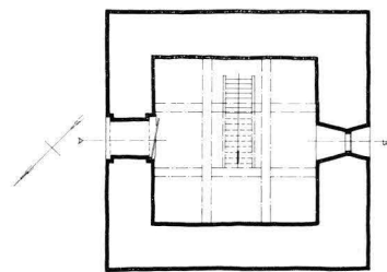
11. TAPULIN KAAKKOISSUUNTAINEN PYSTYLEIKKAUS JA POHJAPIIRROS, 1:300. Snitt av stapeln mot sydöst samt plan, 1:300.
