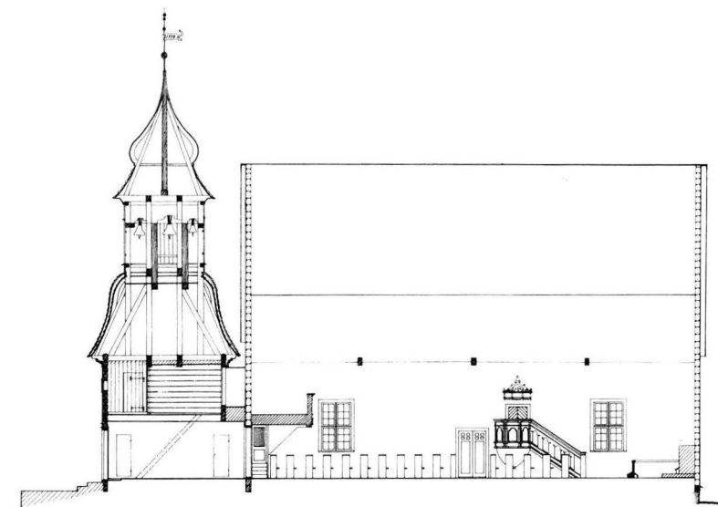
5. KIRKON POHJOISSUUNTAINEN PITKITTÄISLEIKKAUS, 1:300. Längdsnitt av kyrkan mot norr, 1:300.
