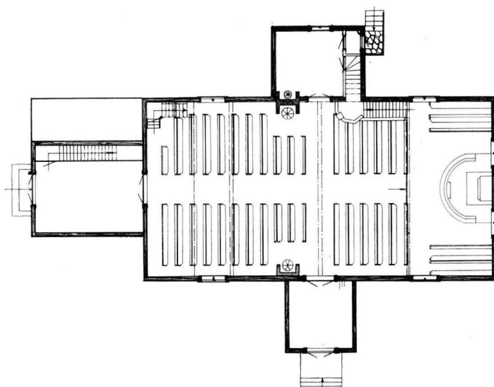
3. KIRKON POHJAPIIRROS, 1:300. Plan av kyrkan, 1:300.
