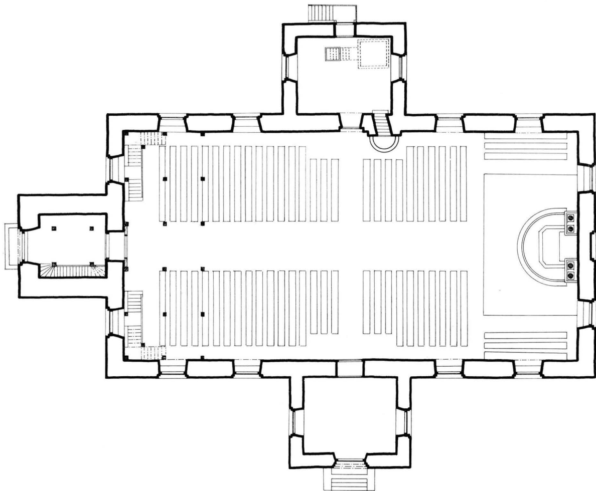
26. KIRKON POHJAPIIRROS, 1:300. Plan av kyrkan, 1:300.
