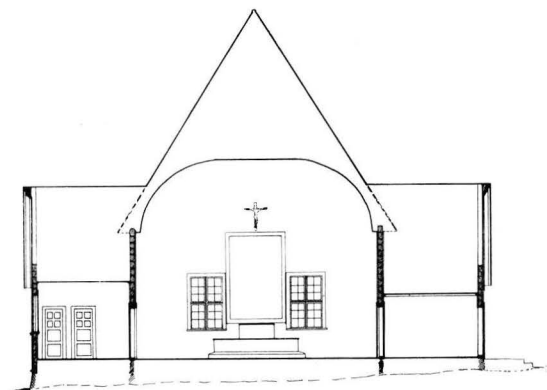
4. KIRKON ITÄSUUNTAINEN POIKITTAIKKAUS, 1:300. Tvärsnitt av kyrkan mot öster, 1:300.
