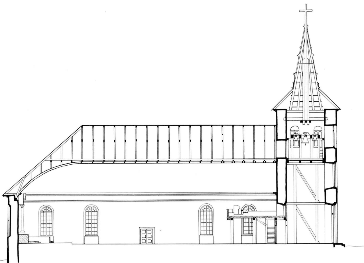
28. KIRKON ETELÄSUUNTAINEN PITKITTÄISLEIKKAUS, 1:300. Längdsnitt av kyrkan mot söder, 1:300.
