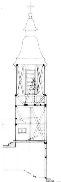
50. TORNIN PYSTYLEIKKAUS, 1:300. Snitt av tornet, 1:300.
