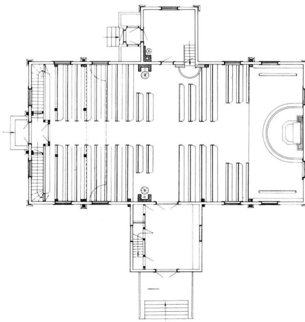
8. KIRKON POHJAPIIRROS, 1:300.
