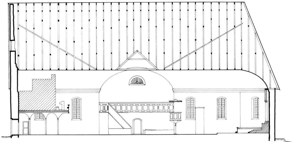
16. KIRKON POHJOISSUUNTAINEN PITKITTÄISLEIKKAUS, 1:300. Längdsnitt av kyrkan mot norr, 1:300.
