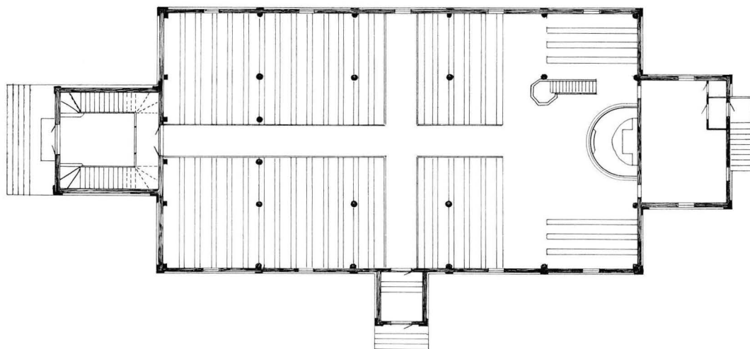
8. KIRKON POHJAPIIRROS, 1:300. Plan av kyrkan, 1:300.
