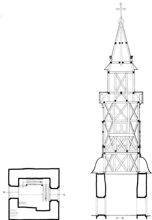
4. KELLOTAPULIN PYSTYLEIKKAUS JA POHJA, 1:300.
