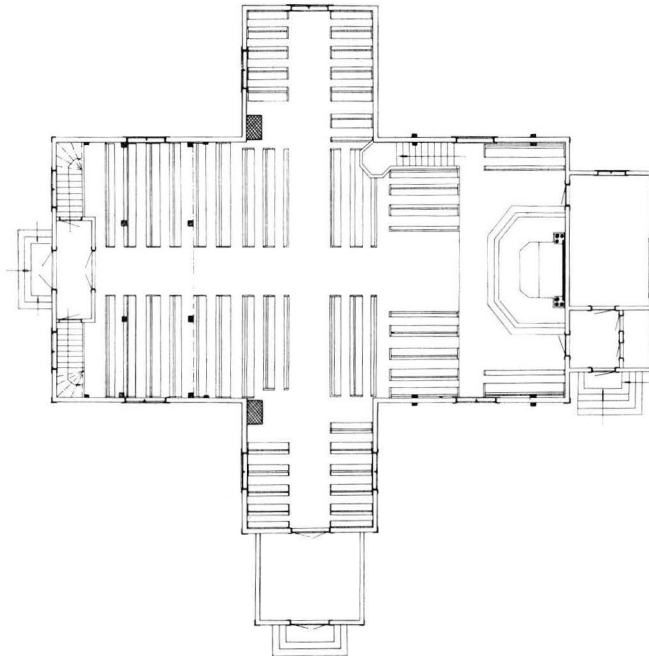
4. KIRKON POHJAPIIRROS, 1:300. Plan av kyrkan, 1:300.
