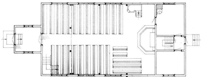
4. KIRKON POHJAPIIRROS, 1:300. Plan av kyrkan, 1:300.
