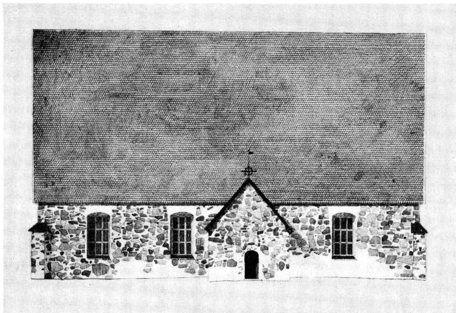
14. KIRKKO ASEHUONEINEEN ETELÄSTÄ, 1:300. Kyrka och vapenhus från söder, 1:300.
