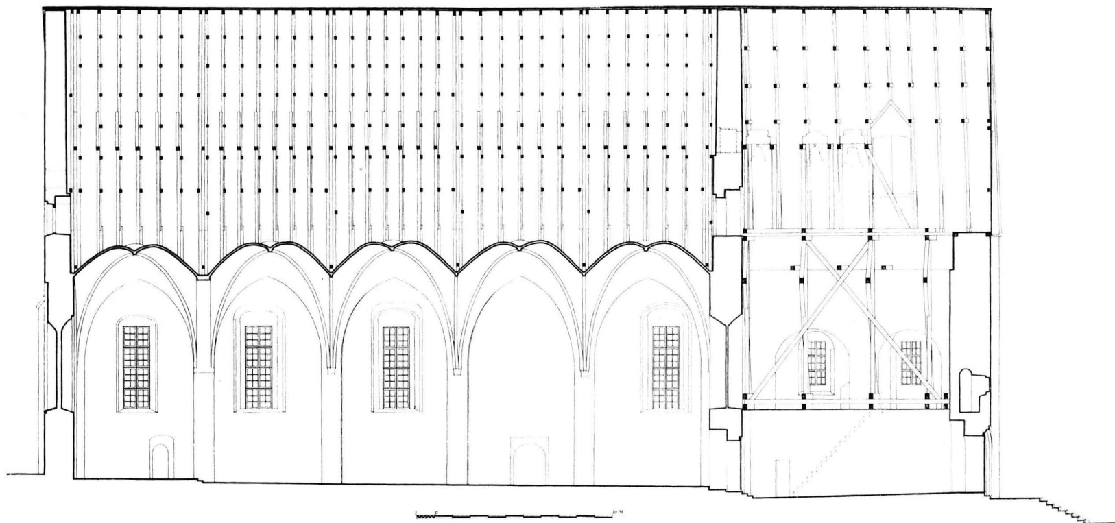
5. KIRKON ETELÄSUUNTAINEN PITKITTÄISLEIKKAUS, 1:300. PIIRUSTUS LAADITTU ENNEN VV. 1959-60 SUORITETTUIJA KORJAUKSIA. Längdsnitt av kyrkan mot söder, 1:300. Ritningen gjord före ändringarna år 1959-60.
