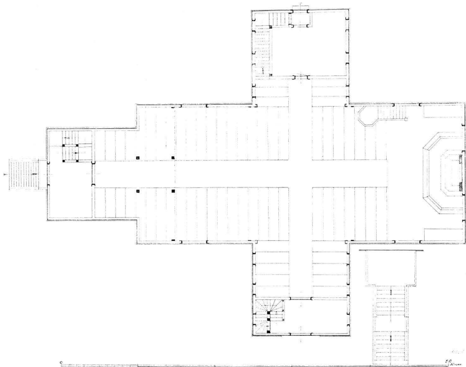
5. KIRKON POHJAPIIRROS, 1:300. Plan av kyrkan, 1:300.
