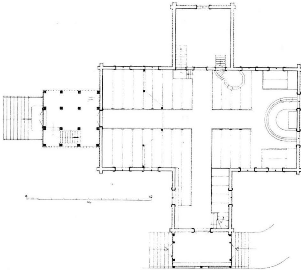
6. KIRKON POHJAPIIRROS, 1:300. Plan av kyrkan, 1:300.
