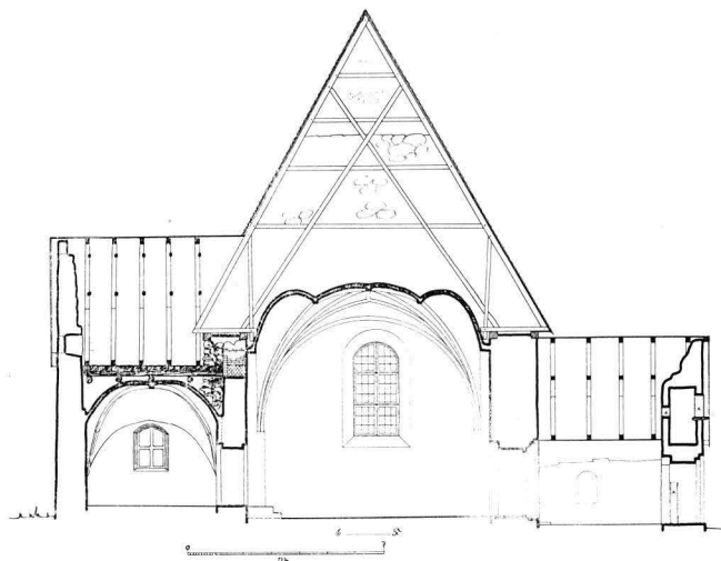
4. KIRKON ITÄSUUNTAINEN POIKITTÄISLEIKKAUS, 1:300. Tvärnitt mot öst av kyrkan, 1:300.
