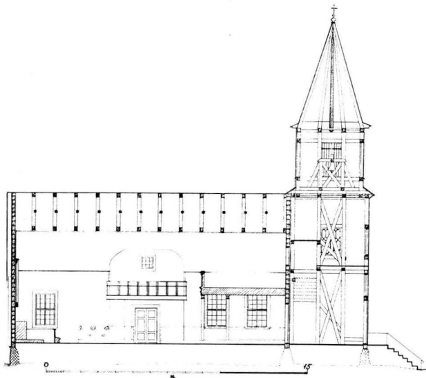
7. RUNKOHUONEEN POHJOISSUUNTAINEN PITKITTÄISLEIKKAUS, 1:300. Längdsnitt av långhuset mot norr, 1:300.
