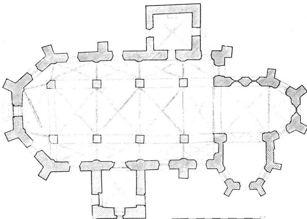
7. KIRKON POHJAPIIRROS, 1:300. Plan av kyrkan, 1:300.
