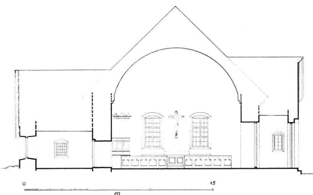
7. RUNKOHUONEEN ITÄSUUNTAINEN POIKITTAISLEIKKAUS, 1:300.
