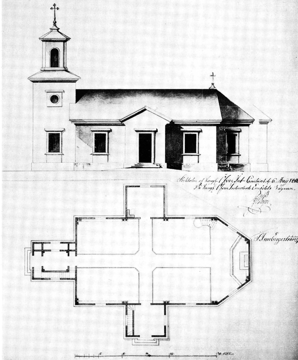
2. S. J. v. ENGSTRÖMIN TEKEMÄT KARJALAN KIRKON PIIRUSTUKSET V:LTÄ 1800. S. J. v. Engeströms ritning till Karjala kyrka år 1800.
