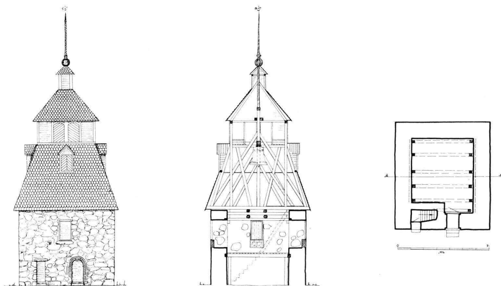
3. TAPULIN ITÄSIVU, LÄNSISUUNTAINEN PYSTYLEIKKAUS JA POHJAPIIRROS, 1:300. Stapelns östside, snitt mot väst och plan, 1:300.
