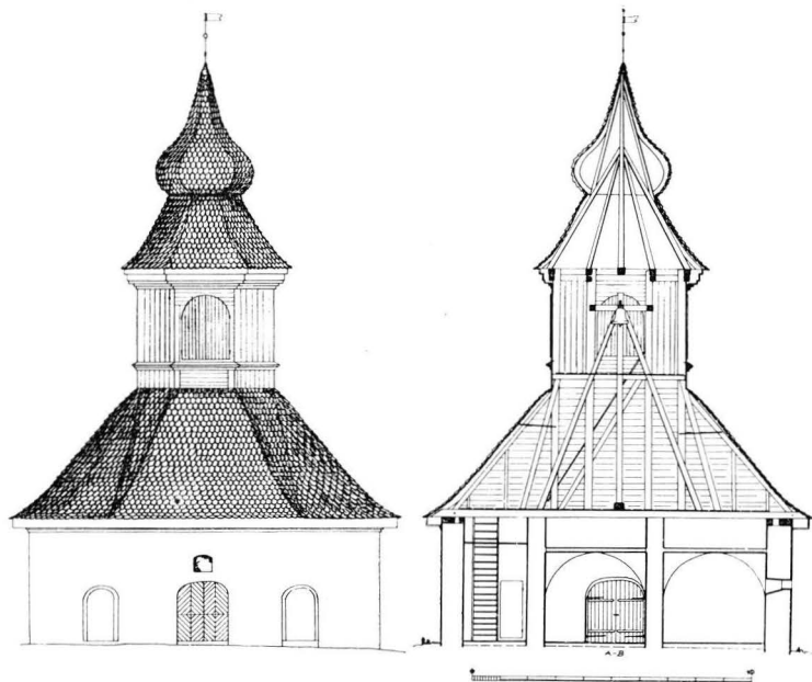
5. TAPULIN LÄNSISIVU JA ITÄSUUNTAINEN PYSTYLEIKKAUS, 1:300. Stapelns västsida och snitt mot öst, 1:300.
