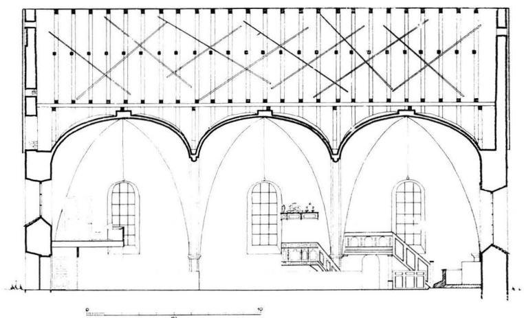
8. RUNKOHUONEEN POHJOISSUUNTAINEN PITKITTÄISLEIKKAUS, 1:300. Längdsnitt av långhuset mot nord, 1:300.
