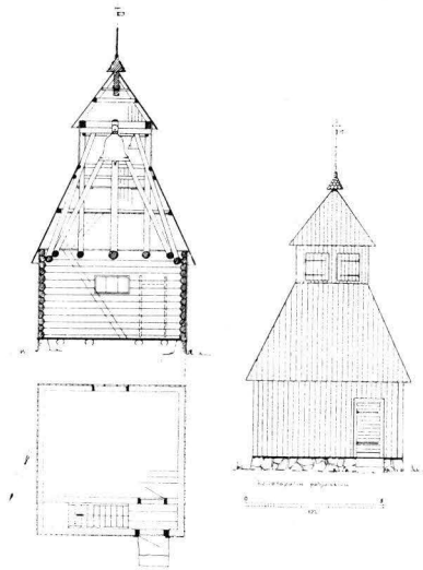
3. TAPULIN ETELÄSUUNTAINEN PYSTYLEIKKAUS, POHJOISSIVU JA POHJAPIIRROS, 1:300. Stapelsnitt mot söder, nordsida och plan, 1:300.
