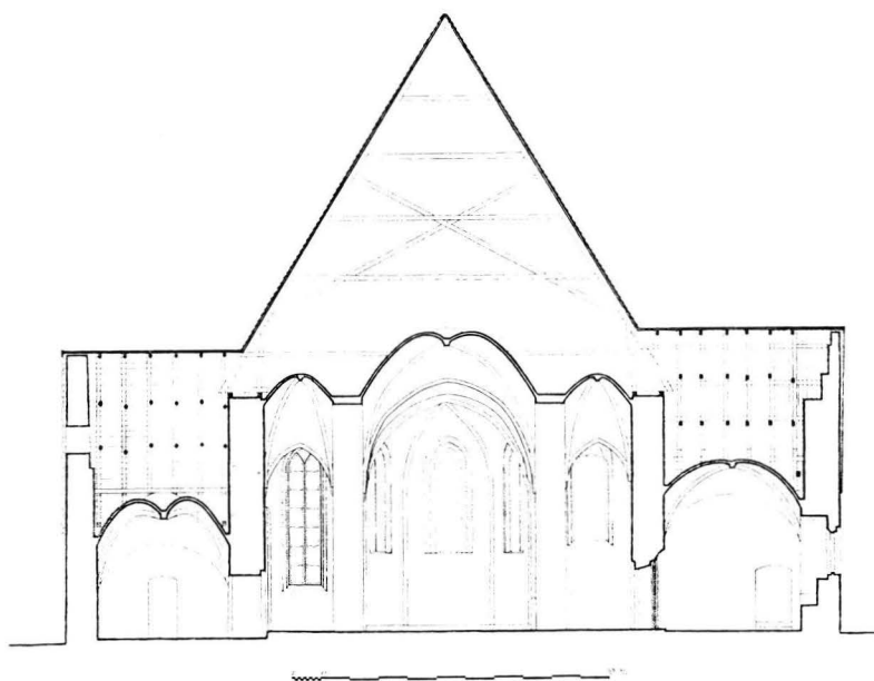
6. KIRKON ITÄSUUNTAINEN POIKITTAIKKAUS, 1:300. Tvärssnitt av kyrkan mot öst, 1:300.
