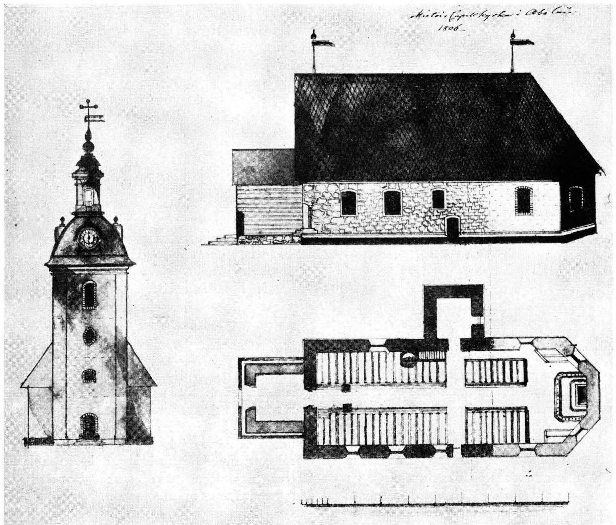
8. JAAKKO GRANDELLIN EHDOTUS MIETOISTEN KIRKON LAAJENTAMISEKSI v. 1806. Jakob Grandells förslag till utvidgning av Mietois kyrka år 1806.
