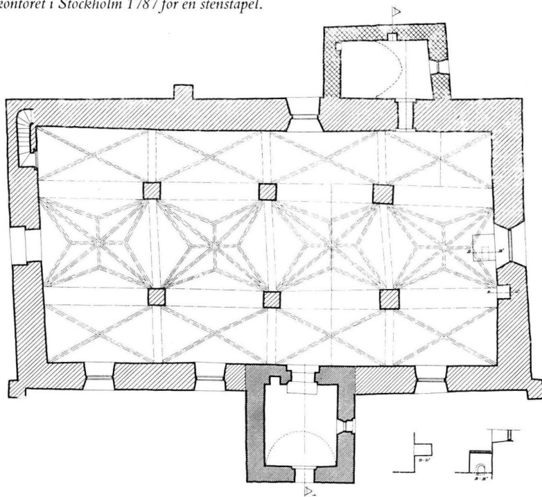
7. KIRKON POHJAPIIRROS, 1:300. Plan av kyrkan, 1:300.
