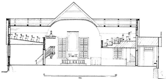
8. KIRKON ITÄSUUNTAINEN POIKITTÄISLEIKKAUS, 1:300. Tvärssnitt av kyrkan mot öst, 1:300.
