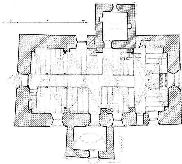
5. KIRKON POHJAPIIRROS, 1:300. Plan av kyrkan, 1:300.
