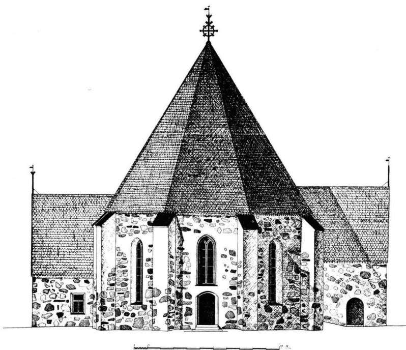
10. LÄNSIKUORI, 1:300. Västkoret, 1:300.
