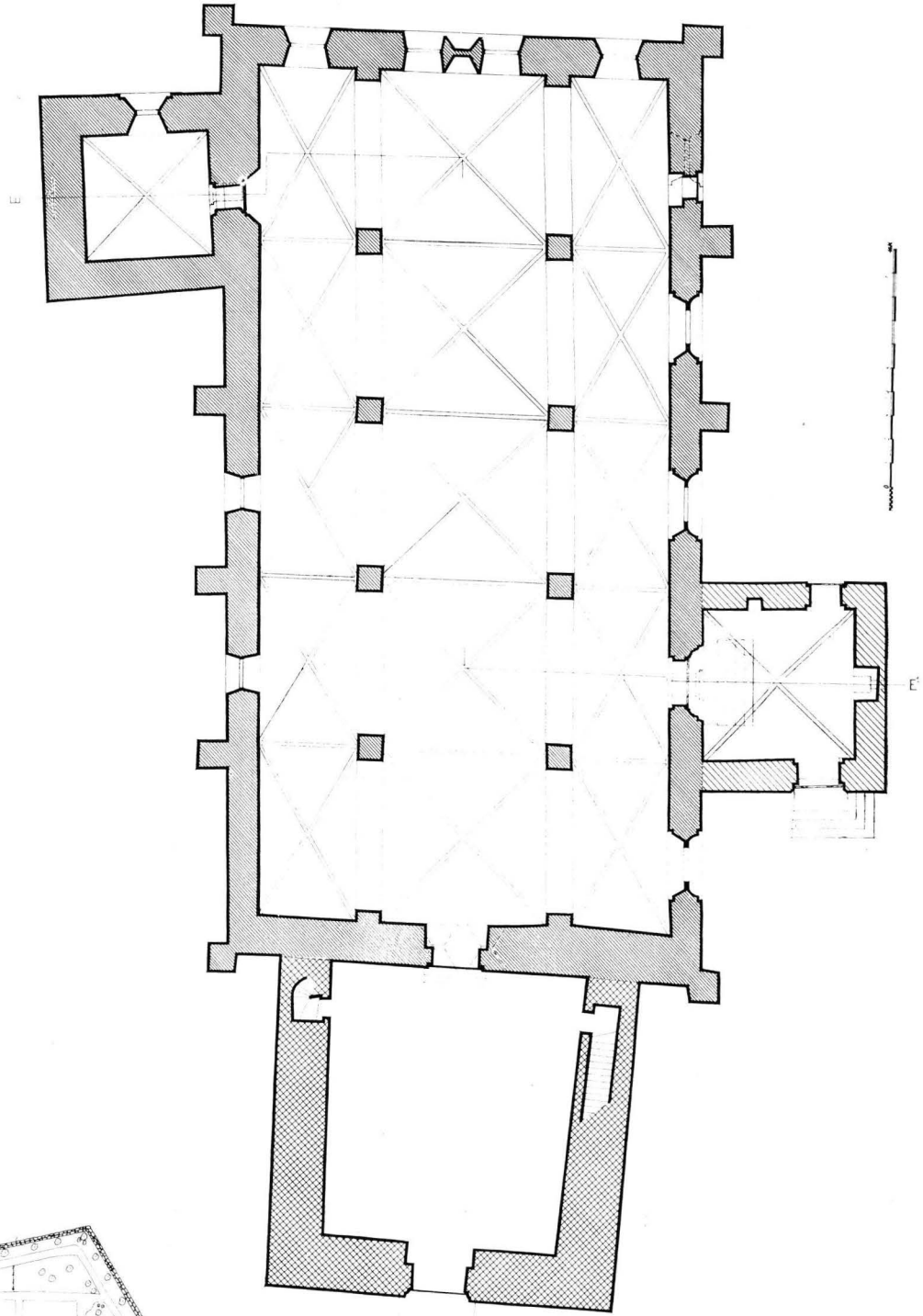
4. KIRKON POHJAPIIRROS, 1:300. Plan av kyrkan, 1:300.
