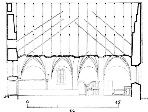
7. RUNKOKUONEEN POHJOISSUUNTAINEN PITKITTÄISLEIKKAUS, 1:300. Längdsnitt av långhuset mot norr, 1:300.
