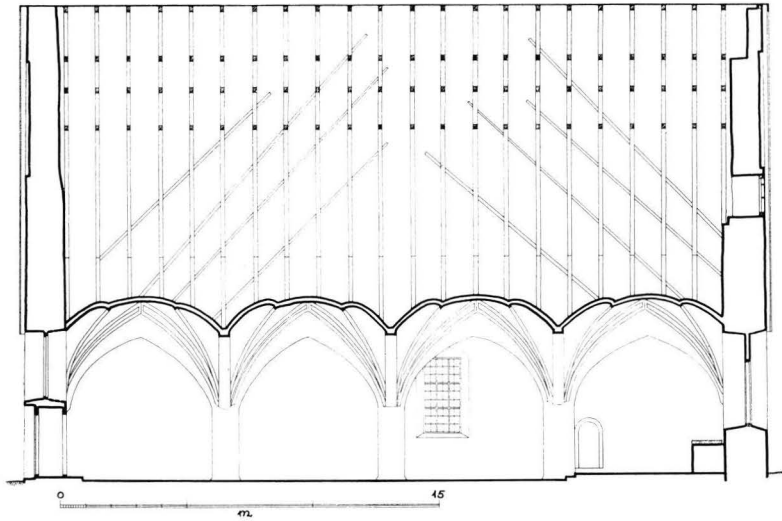
8. RUNKOHUONEEN POHJOISSUUNTAINEN PITKITTÄISLEIKKAUS, 1:300. Längdsnitt av långhuset mot nord, 1:300.
