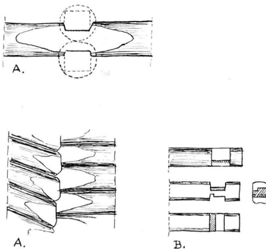
9. TORNIN NURKKASALVOS. Tornets knuttimring.
