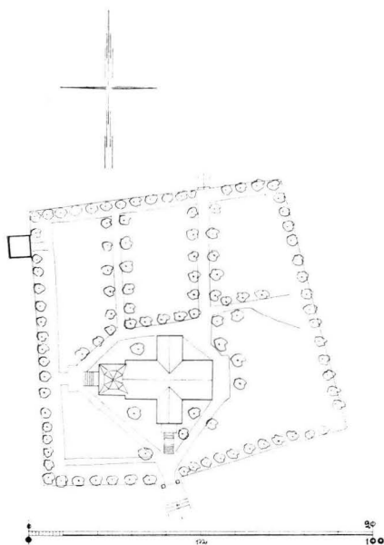
2. ASEMAPIIRROS, 1:2000. Situationsplan, 1:2000.
