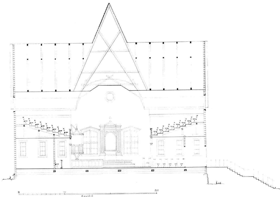
4. KIRKON ITÄSUUNTAINEN POIKITTÄISLEIKKAUS, 1:300. Tvärnitt av kyrkan mot öst, 1:300.
