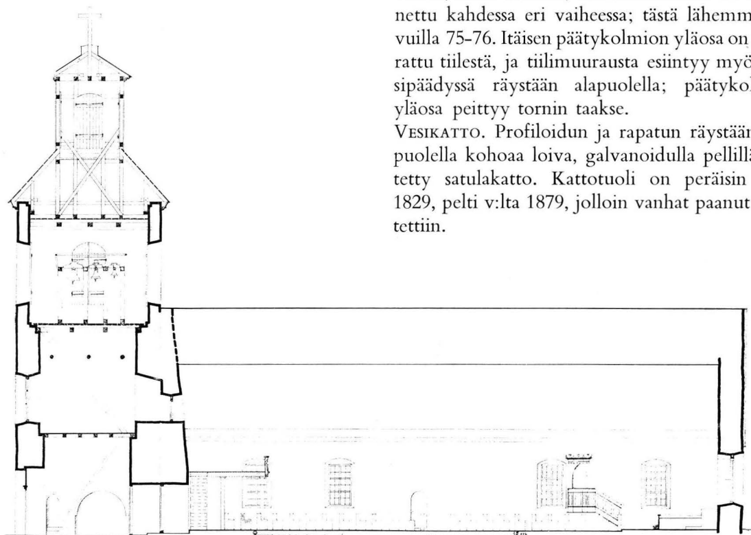
5. RUNKOHUONEEN POHJOISSUUNTAINEN PITKITTÄISLEIKKAUS, 1:300. Längdsnitt mot norr av långhuset, 1:300.
