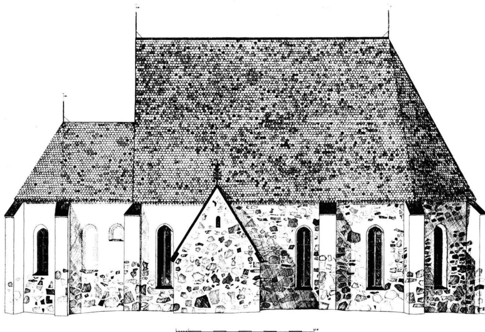
9. KIRKON POHJOISSIVU, 1:300. Nordfasad, 1:300.
