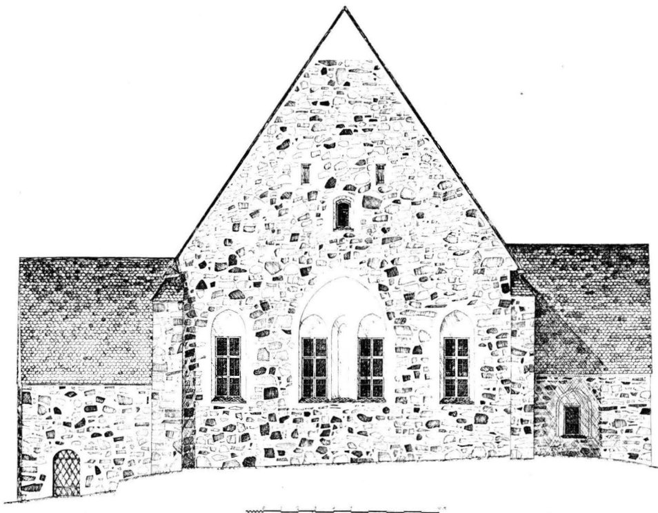
17. KIRKON ITÄSIVU, 1:300. PIIRUSTUS LAADITTU ENNEN V:TA 1959. Kyrkans östsida, 1:300. Ritningen utförd före år 1959.
