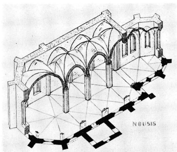
16. ENSIMMÄINEN HOLVAUS RINGBOMIN REKONSTRUOINNIN MUKAAN. Ringboms rekonstruktion av de första valven.
