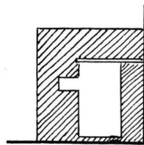
13. PÄÄALTтарIN PYSTYLEIKKAUS, 1:60. Lodrätt snitt genom huvudaltaret, 1:60.
