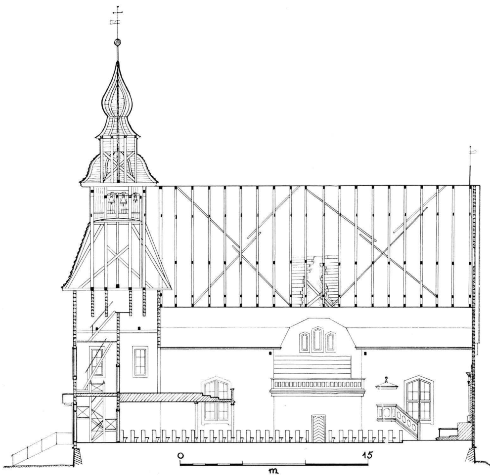
3. RUNKOHUONEEN JA TORNIN PÖHJOISSUUNTAINEN PITKITTÄISLEIKKAUS, 1:300. Längdsnitt mot norr av långhus och torn, 1:300.
