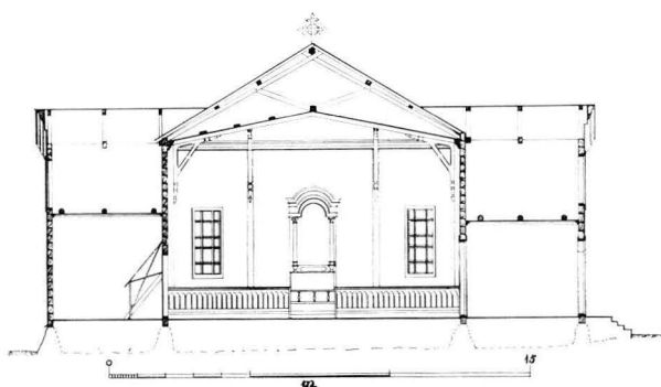
7. KIRKON POHJOISSUUNTAINEN PITKITTÄISLEIKKAUS, 1:300. Längdsnitt av kyrkan mot norr 1:300.
