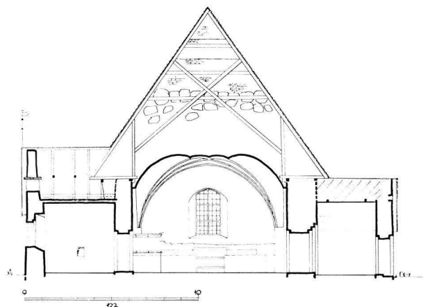
6. KIRKON ITÄSUUNTAINEN POIKITTÄISLEIKKAUS, 1:300. Tvärssnitt av kyrkan mot öst, 1:300.
