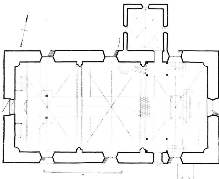
7. KIRKON POHJAPIIRROS, 1:300. Plan av kyrkan, 1:300.
