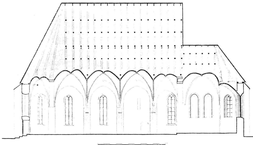
8. RUNKOHUONEEN POHJOISSUUNTAINEN PITKITTÄISLEIKKAUS, 1:300.
