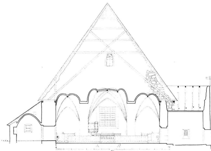
9. KIRKON ITÄSUUNTAINEN POIKITTÄISLEIKKAUS, 1:300. Tvärnsnitt av kyrkan mot öst, 1:300.
