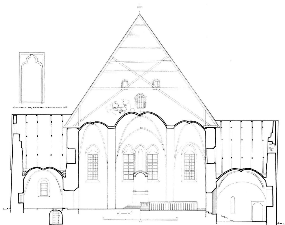
6. KIRKON ITÄSUUNTAINEN POIKITTAISELEIKKAUS, 1:300. PIIRUSTUS LAADITTU ENNEN V. 1959 SUORITETTUA KORJAUSTA, JOLLOIN MM. KUORI-IKKUNA PALAUTETTIIN ALKUPERÄISEEN MUOTOONSAA.
