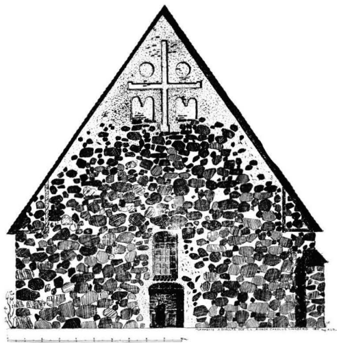
10. KIRKON LÄNSIPÄÄTY, 1:300. Kyrkans västgavel, 1:300.
