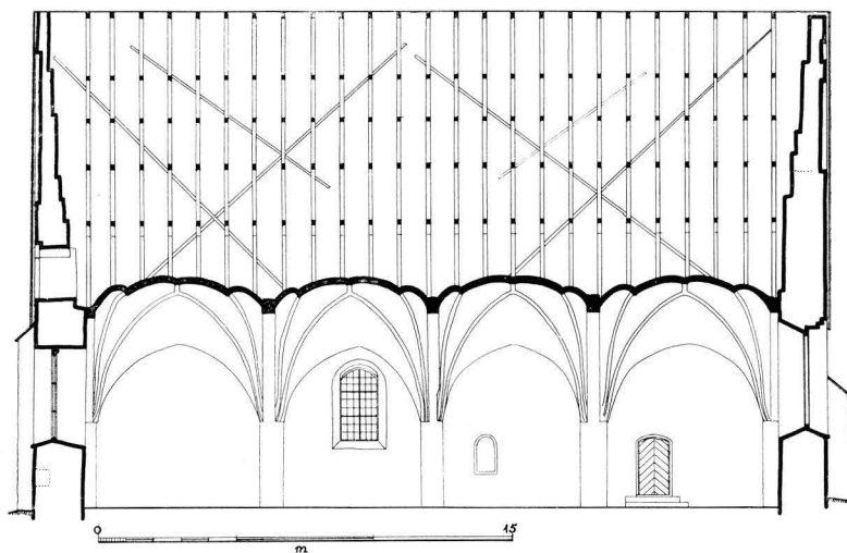
5. RUNKOHUONEEN PÖHJOISSUUNTAINEN PITKITTÄISLEIKKAUS, 1:300. Längdsnitt av långhuset mot norr, 1:300.
