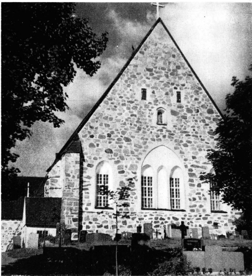
8. ITÄPÄÄTY. VALOKUVA OTETTU ENNEN V. 1959 SUORITETTUA KORJAUSTA. Östgaveln. Foto taget före reparationen år 1959.
