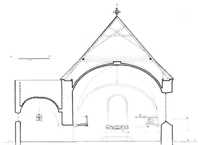
9. KIRKON ITÄSUUNTAINEN POIKITTÄISLEIKKAUS, 1:300. Tvärnsnitt av kyrkan mot öster, 1:300.
