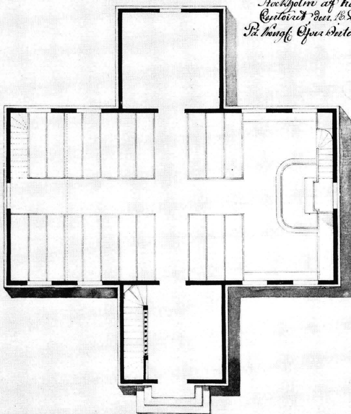
5. S. J. v. ENGSTRÖMIN V. 1800 LAATIMAT PIIRUSTUKSET VAHDON KIRKKOA VARTEN. S. J. v. Engströms ritningar till Vahto kyrka år 1800.
