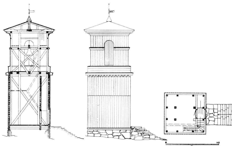
3. TAPULIN ITÄSUUNTAINEN PYSTYLEIKKAUS, LÄNSISIVU JA POHJAPIIRROS, 1:300. Snitt av stapeln mot öst, stapeln västsidan och plan, 1:300.
