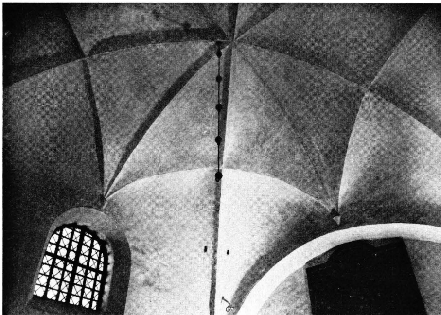
14. KIRKON HOLVEISSA ON RUOTEIDEN ASEMESTA TERÄVÄT TAITEKOHDAT. KUVASSA NÄKYVÄ SAKARISTON TÄHTIHOLVI. Valven har skarpa åser i st. f. ribbor. På bilden sakristians stjärnvalv.
