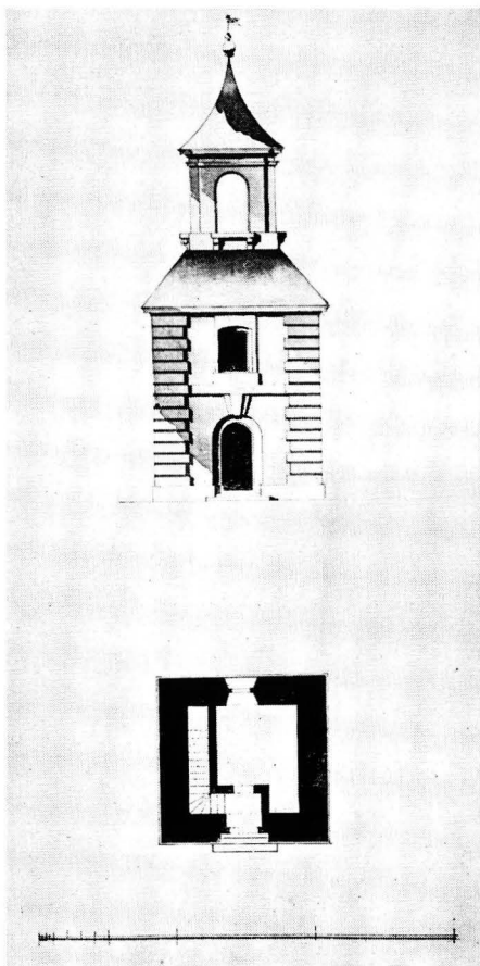
6. TUKHOLMAN INTENDENTTIKONTTORIN V. 1787 PÄIVÄTTY KIVITAPULIA KOSKEVA EDHOTUS. Ritning från intendentkontoret i Stockholm 1787 för en stenstapel.
