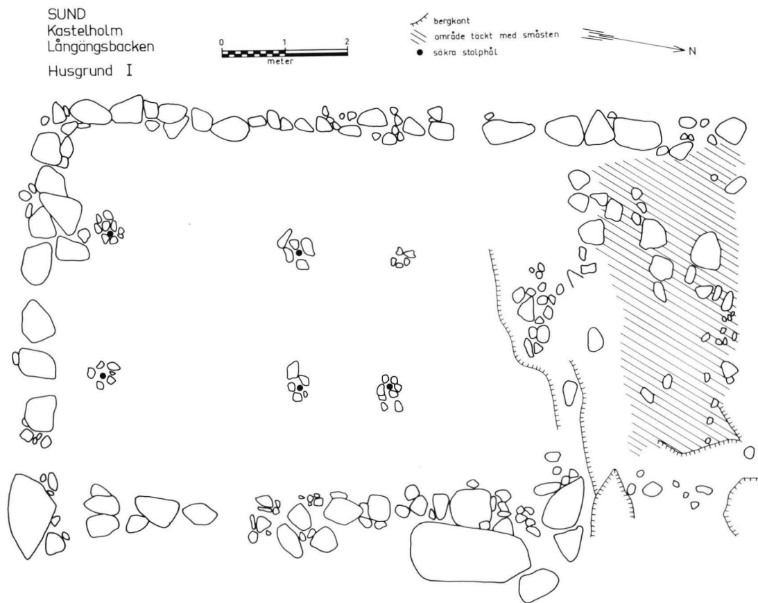
Bild 21. Karta över husgrund I på Långängsbacken.
