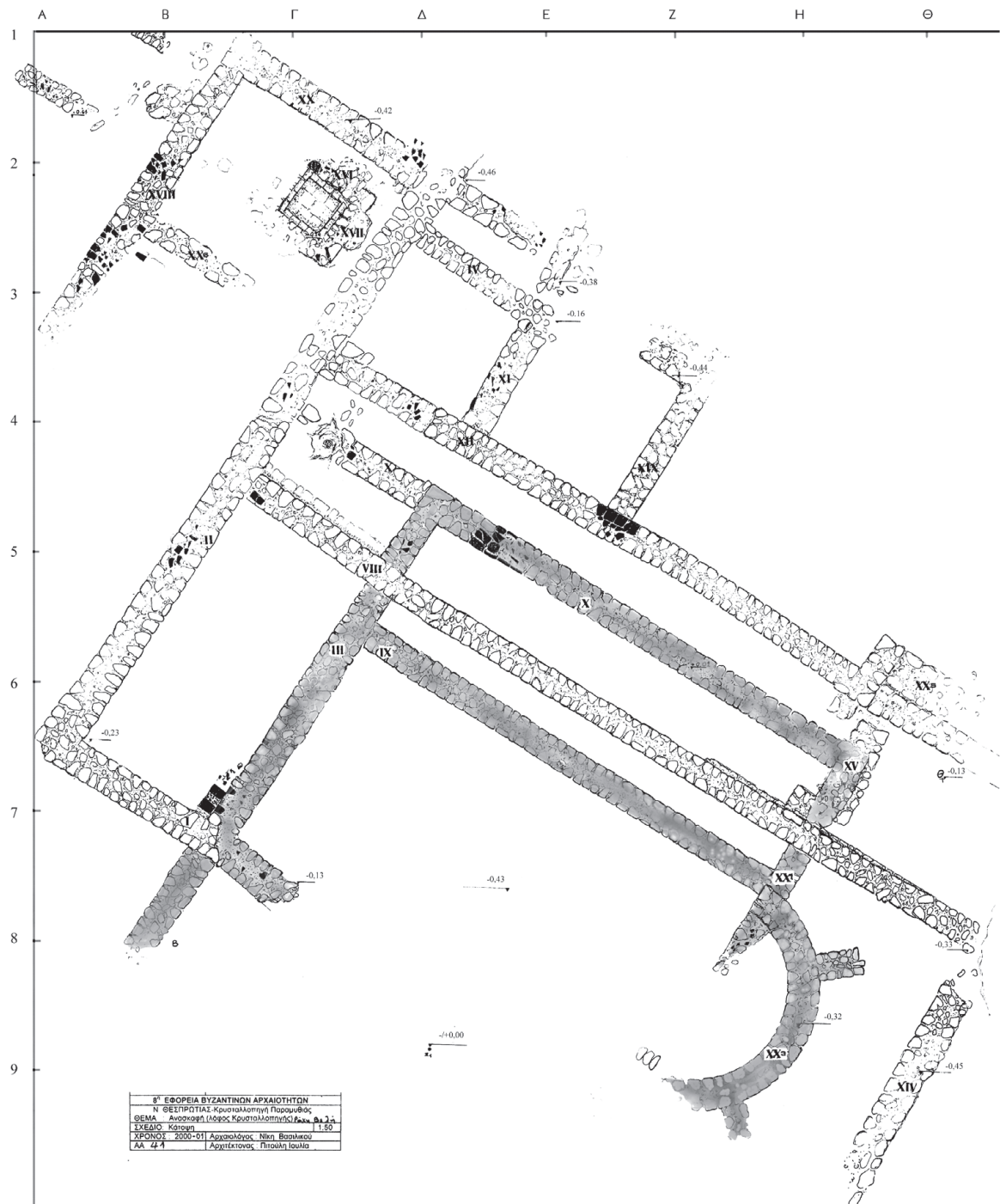
Εικ. 2. Κάτοψη των οικοδομικών λειψάνων.
